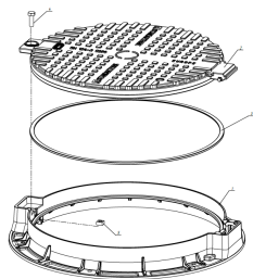
Schema generala montaj
